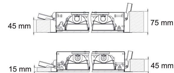
ALBO LEDIZ® M600X600 4 3100/840 DPB DS
