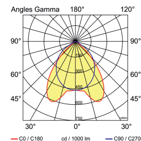
ALBO LEDIZ® M600X600 4 3100/840 DPB DS
